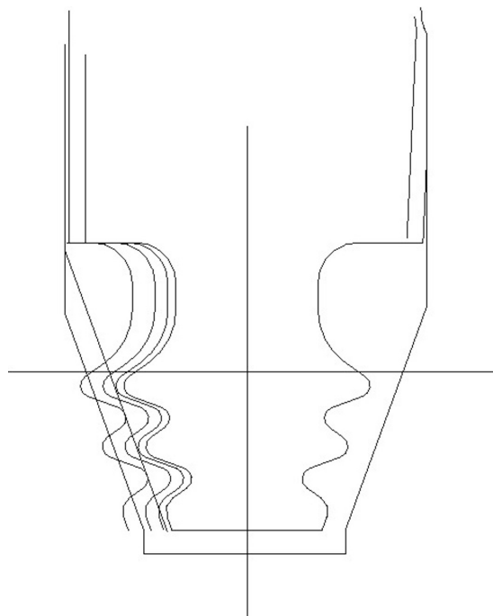
Рис. 3. Схема снимаемых припусков по «ёлке» хвостовика
