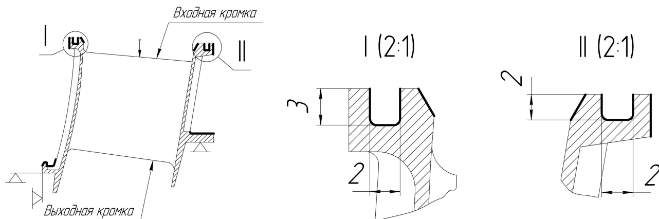
Рис. 1. Обработка со стороны входной кромки
